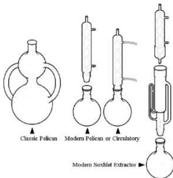
Рисунок 11: Циркуляционная стеклянная посуда
